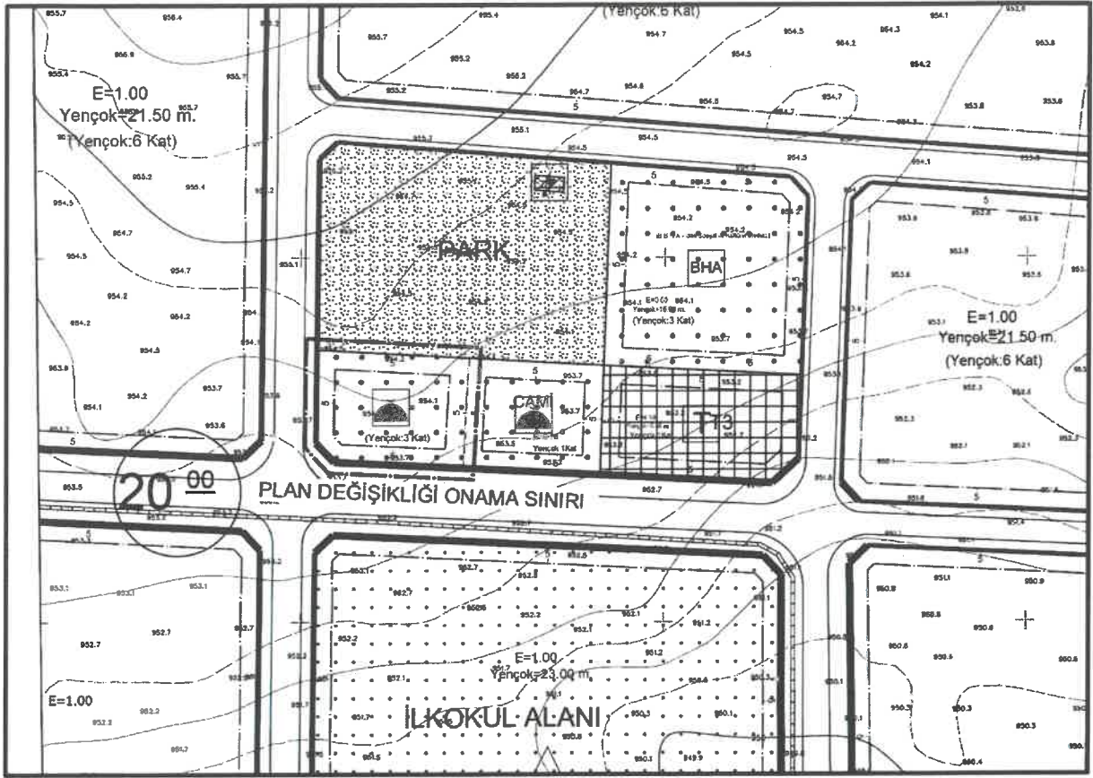
Şekil 2: Yalangöz Planlama Alanı Mevcut 1/1.000 Uygulama İmar Planı
