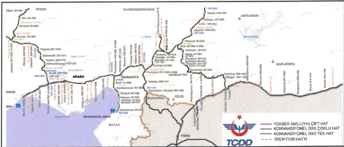
Şekil 4. Gaziantep İli Demiryolu Ağı
