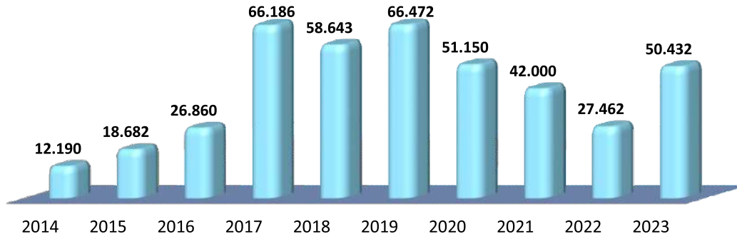
Grafik 49 - İmalatı Yapılan Boru Miktarları(m)
