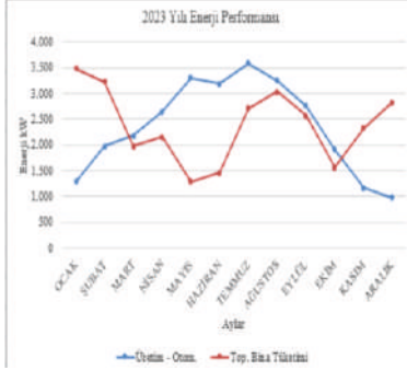
Grafik 7 - 2023 Yılı Enerji Performansı
