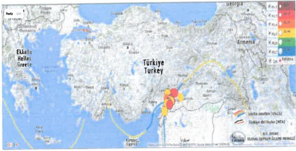
Harita 51: 1916'den günümüze Gaziantep ve yakın çevresinde meydana gelen depremler (TUDİM) ve çalışma alanı ve çevresi diri kırıkları verilmiştir.
