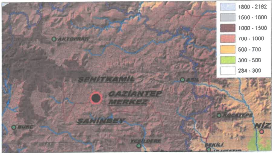
Harita 43 : İnceleme Alanı Ve Çevresi Yükselti Kuşakları Haritası
