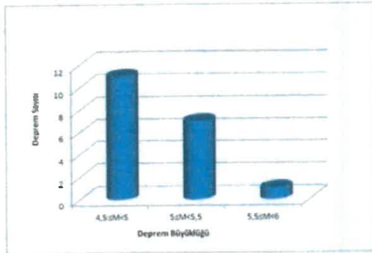
Gaziantep ve çevresi 1900 yılından günümüze kadar olmuş deprem sayısı – deprem büyüklüğü ( M > 4.5 ) arasındaki ilişkiyi gösterir histogram.
