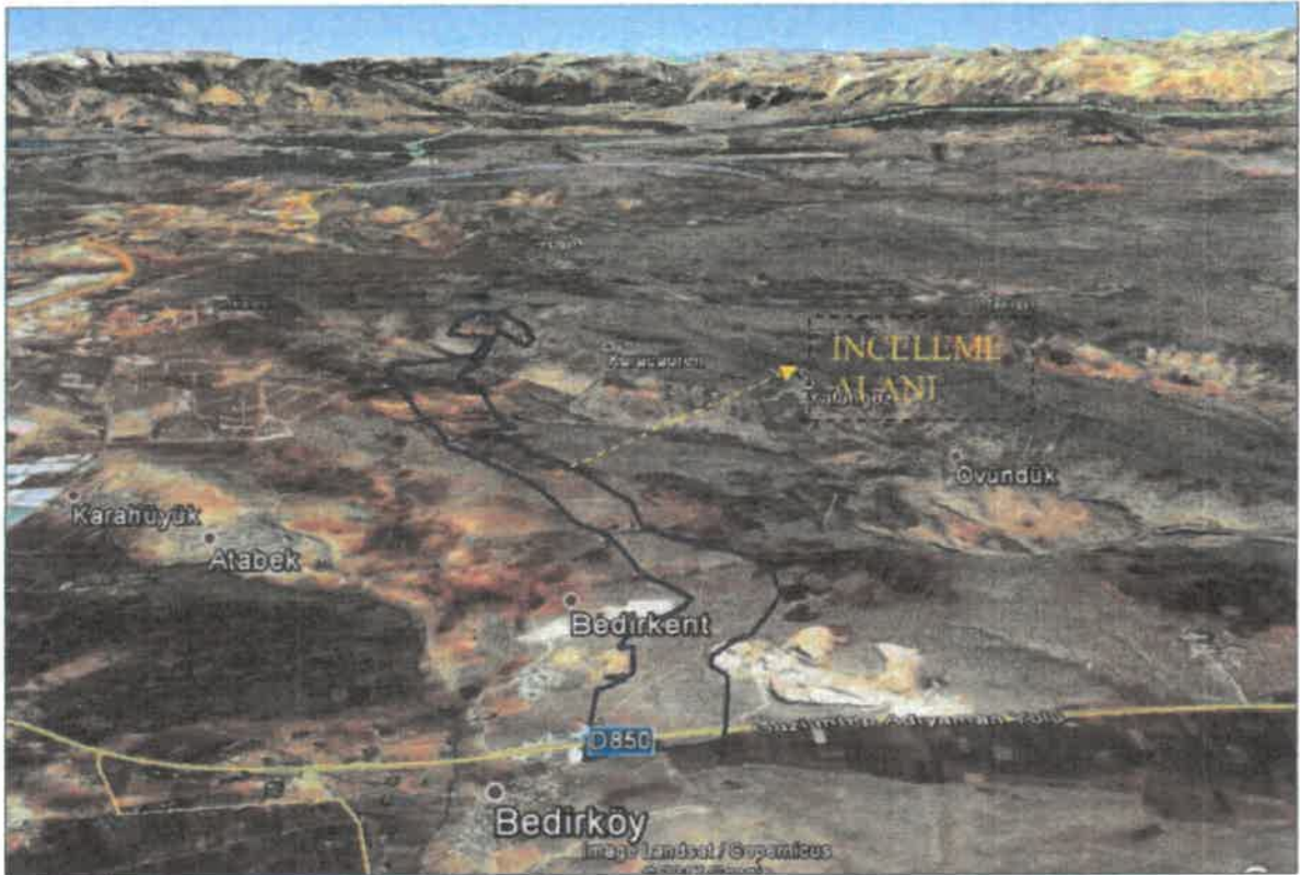
Harita 45: İnceleme Alanı Jeomorfolojisini Gösteren Genel Görünüm
