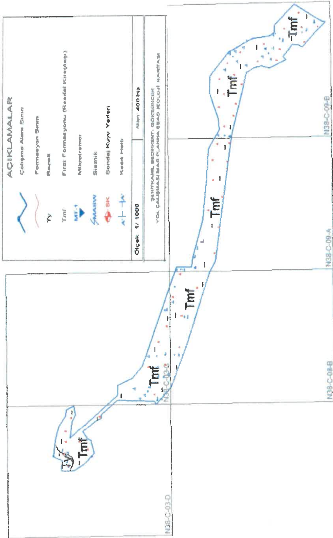
Harita 49: İnceleme Alanı Jeoloji Haritası
