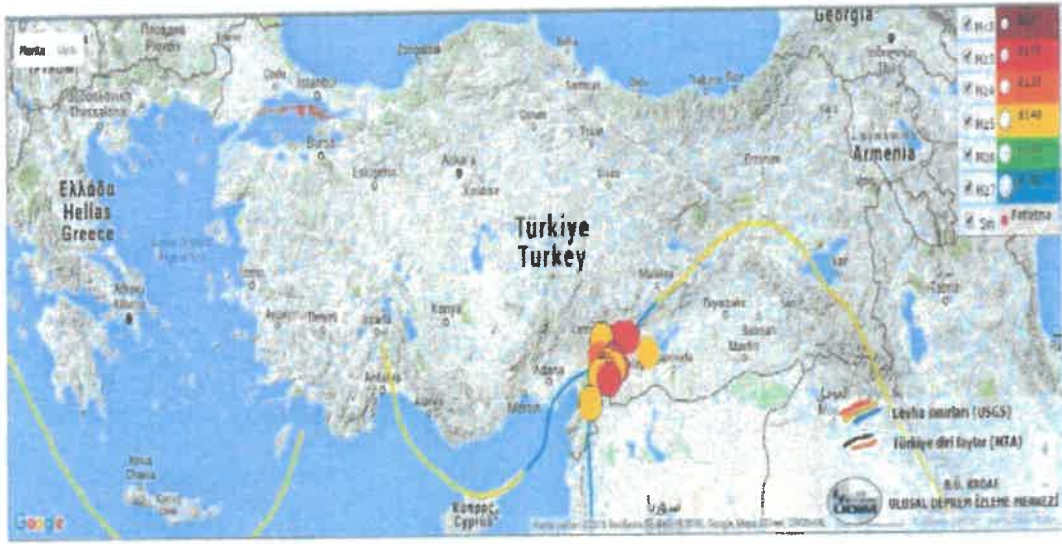
Harita 52: 1916'dan günümüze Gaziantep ve yakın çevresinde meydana gelen depremler (UDİM) ve çalışma alanı ve çevresi diri kırıkları verilmiştir.
