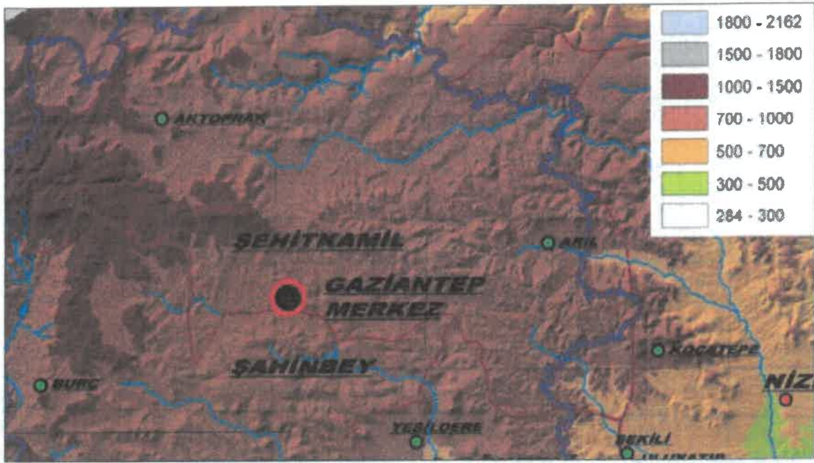
Harita 44: İnceleme Alanı ve Çevre Yükselti Kuşakları Haritası
