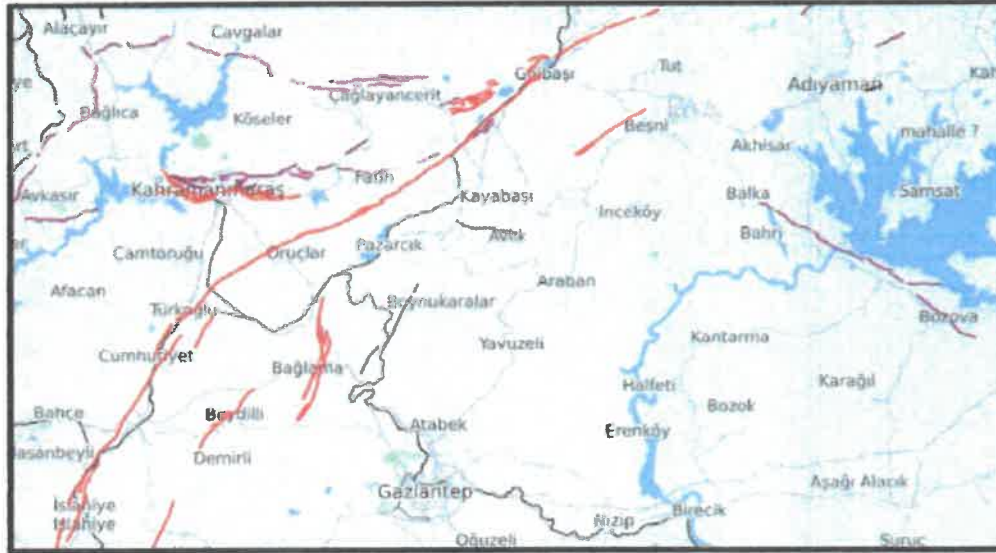
Harita 54: Gaziantep ve Çevresi Yenilenmiş Diri Fay Haritası (M.T.A)
