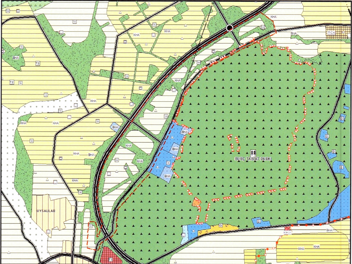
Şekil 9: Çamtepe ve Cebeler Mahalleleri Proje Alanı Mevcut 1/25000 Ölçekli Nazım İmar Planı
