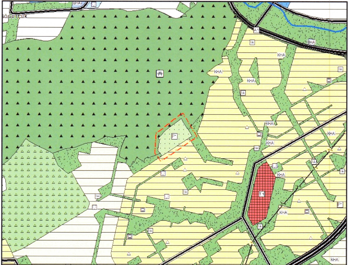
Şekil 5: Gazitepe Mahallesi Proje Alanı Öneri 1/25000 Ölçekli Nazım İmar Planı
