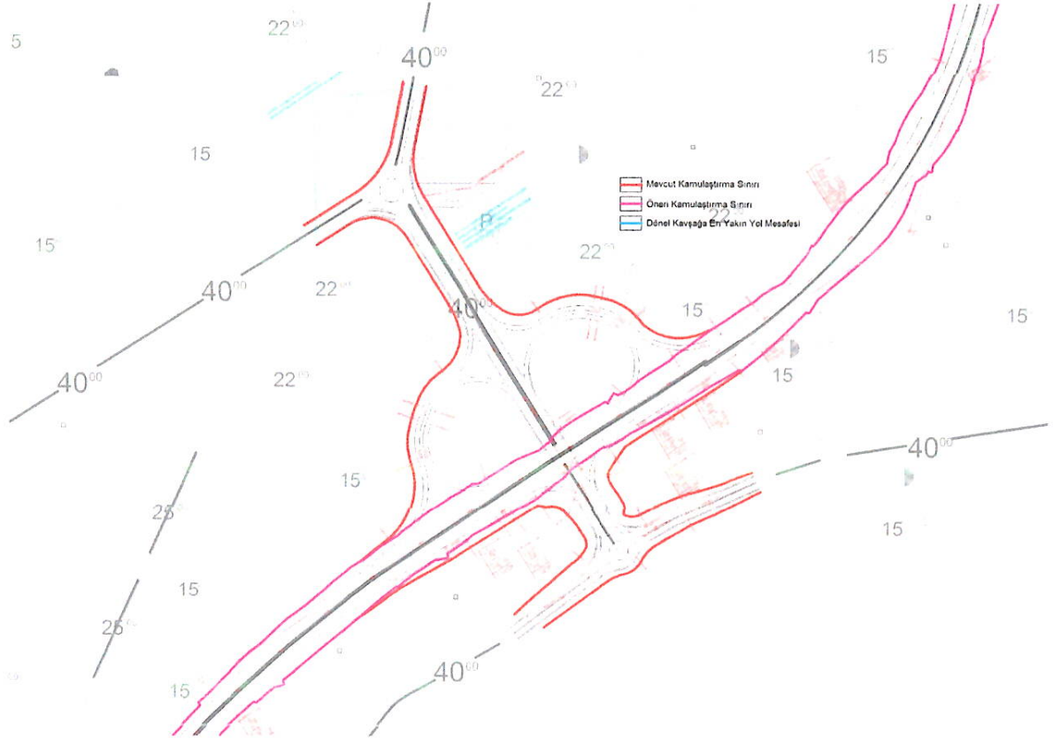
Şekil 3: Değişen Kamulaştırma Sınırı ve Öneri Kavşak Projesi – Mevcut Nazım İmar Planı
