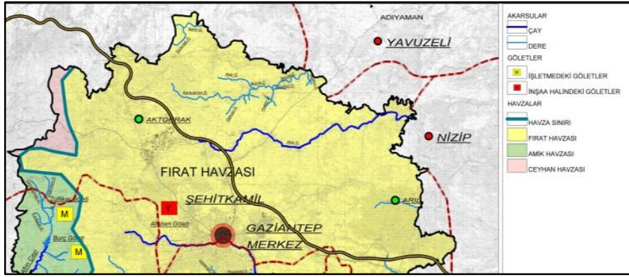
Şekil 13: Hidrolojik Yapı
