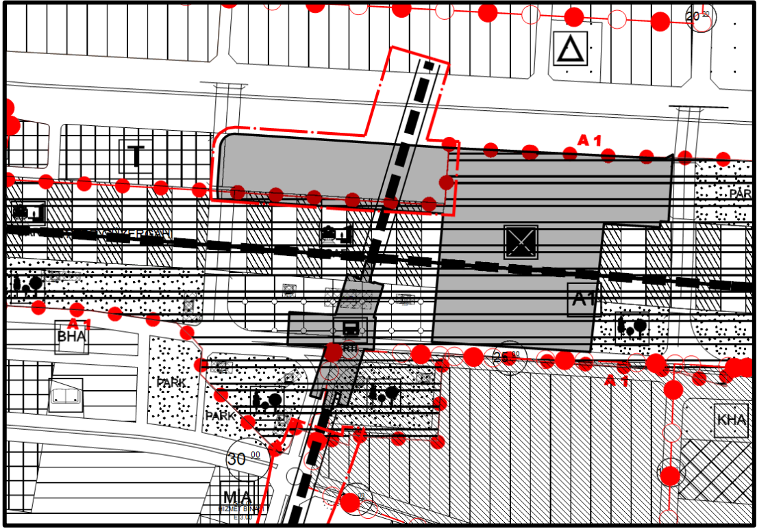
Şekil 16 1/5000 Ölçekli Nazım İmar Planı Değişikliği - Toplu Taşım Türleri Arası Değişim ve Aktarma Alanı ve 1 No'lu Gar İstasyonu
