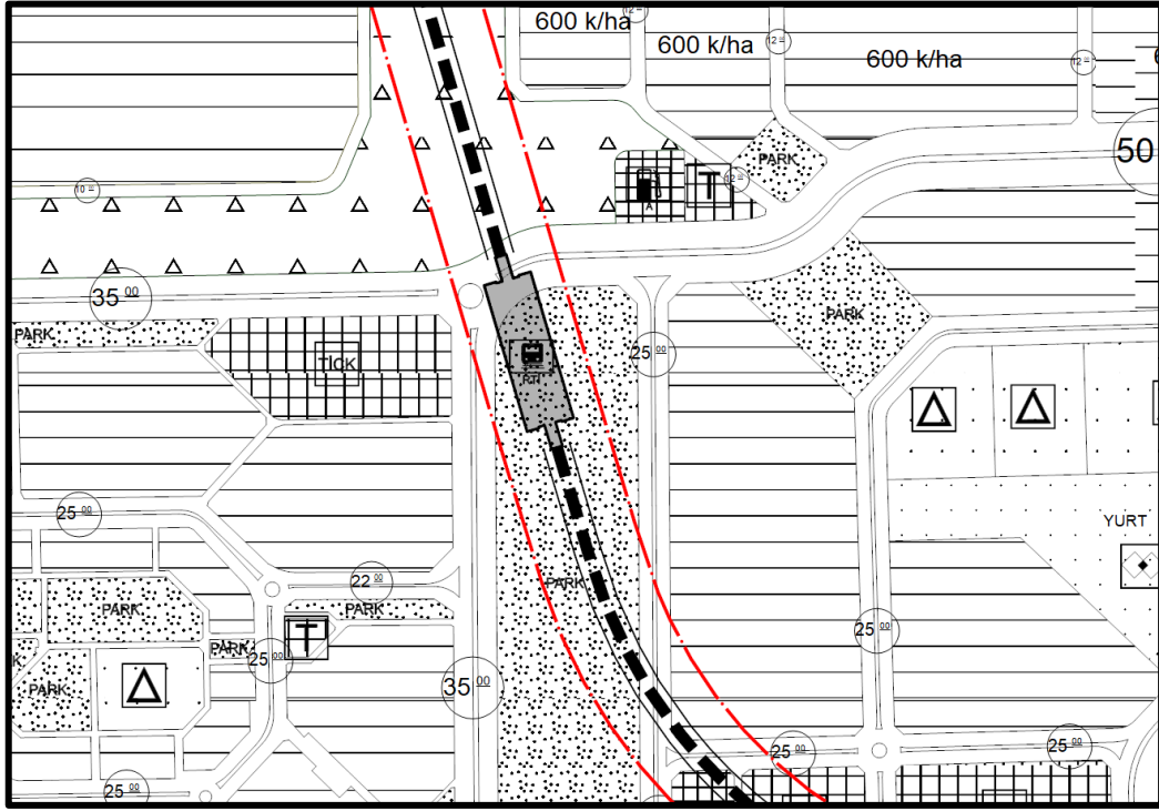
Şekil 22 1/5000 Ölçekli Nazım İmar Planı Değişikliği - 7 No'lu Akkent Parkı İstasyonu
