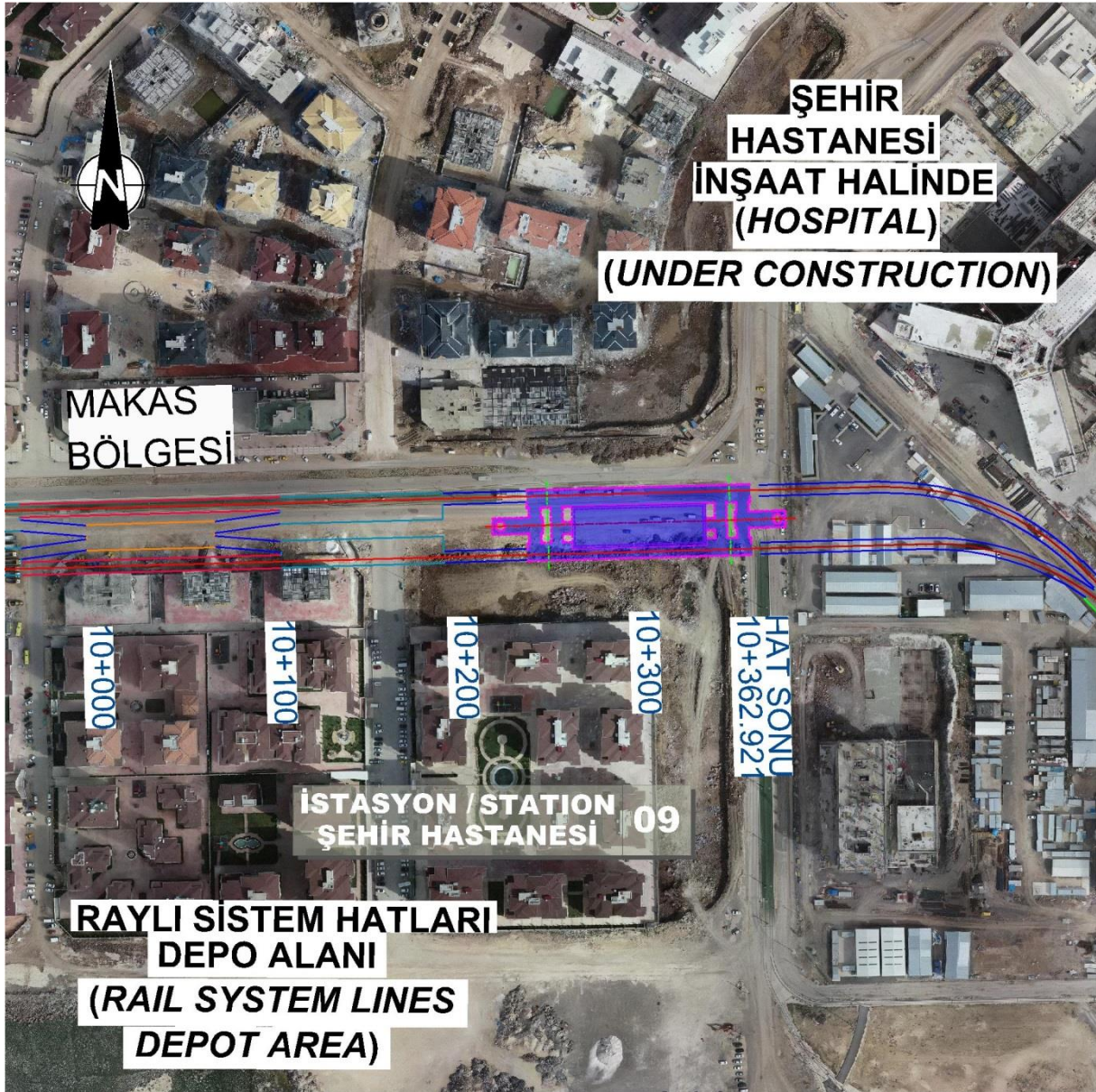
Şekil 12 Şehir Hastanesi İstasyonu
