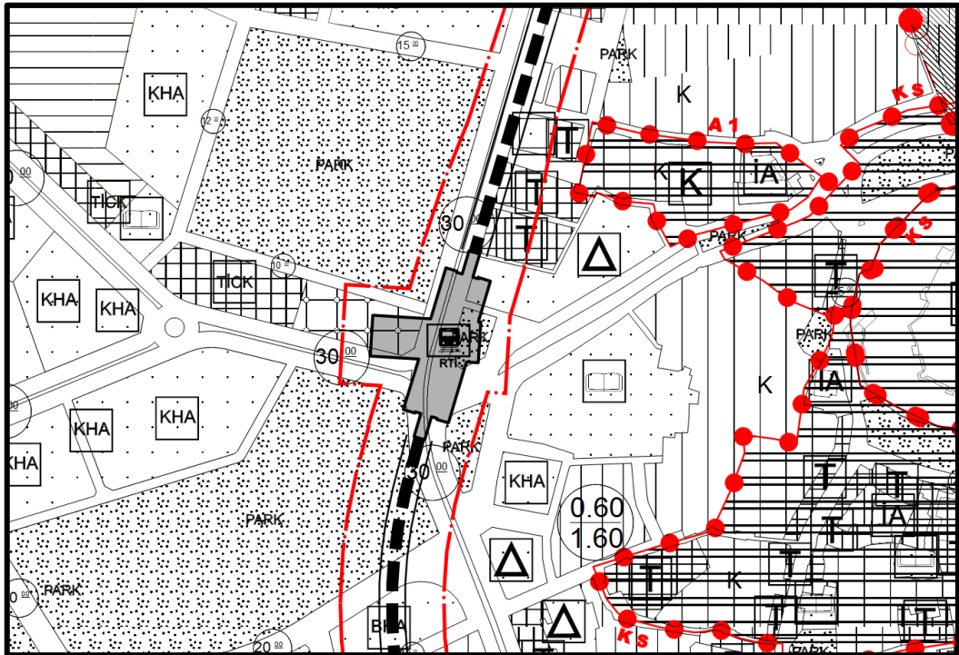
Şekil 17 1/5000 Ölçekli Nazım İmar Planı Değişikliği - 2 No'lu 15 Temmuz Demokrasi Meydanı İstasyonu
