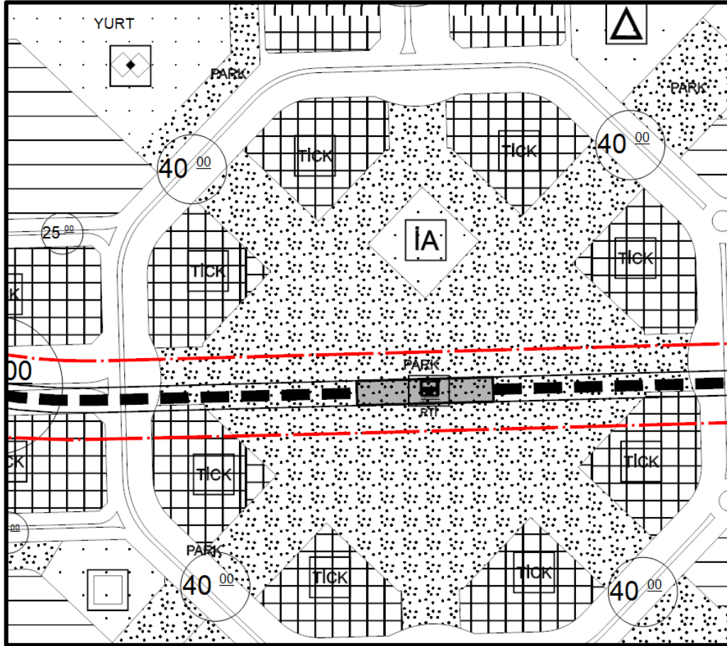
Şekil 23 1/5000 Ölçekli Nazım İmar Planı Değişikliği - 8 No'lu Akkent İstasyonu
