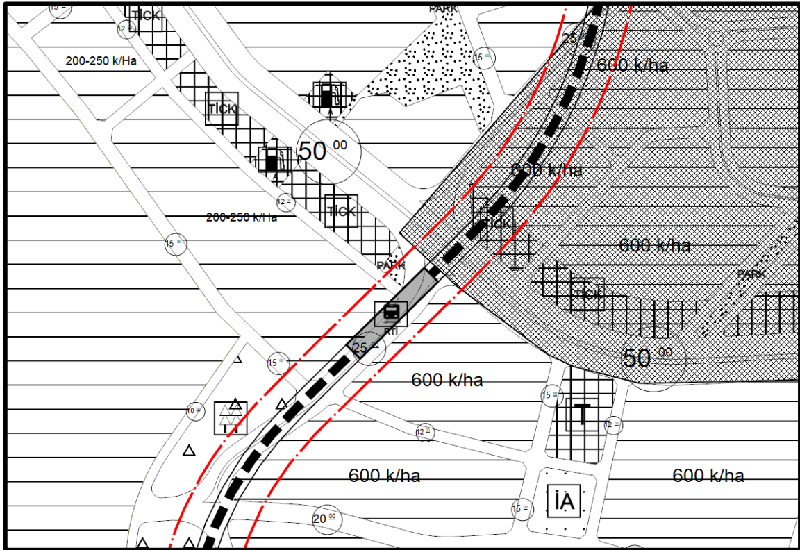
Şekil 21 1/5000 Ölçekli Nazım İmar Planı Değişikliği - 6 No'lu Yeşilvadi İstasyonu
