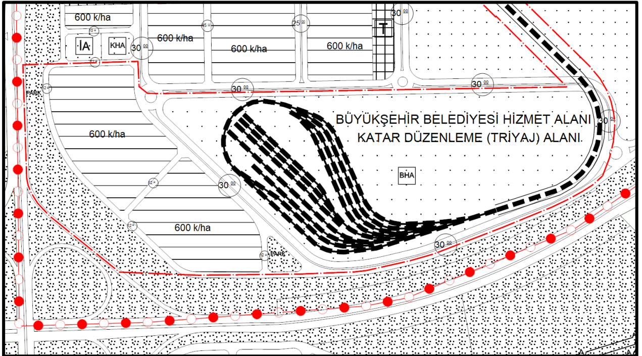
Şekil 25 1/5000 Ölçekli Nazım İmar Planı Değişikliği - Büyükşehir Belediye Hizmet Alanı (Katar Düzenleme (Triyaj) Alanı)
