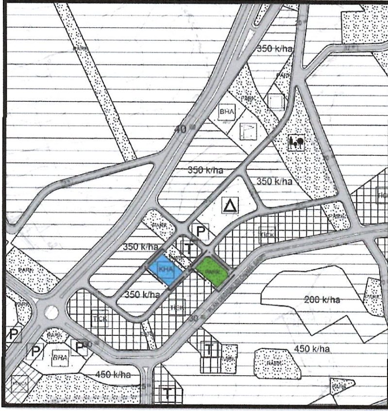
Şekil 5: Şahinbey İlçesi Küçükkızıllıhisar Mahallesi Mevcut 1/5000 Ölçekli Nazım İmar Planı
