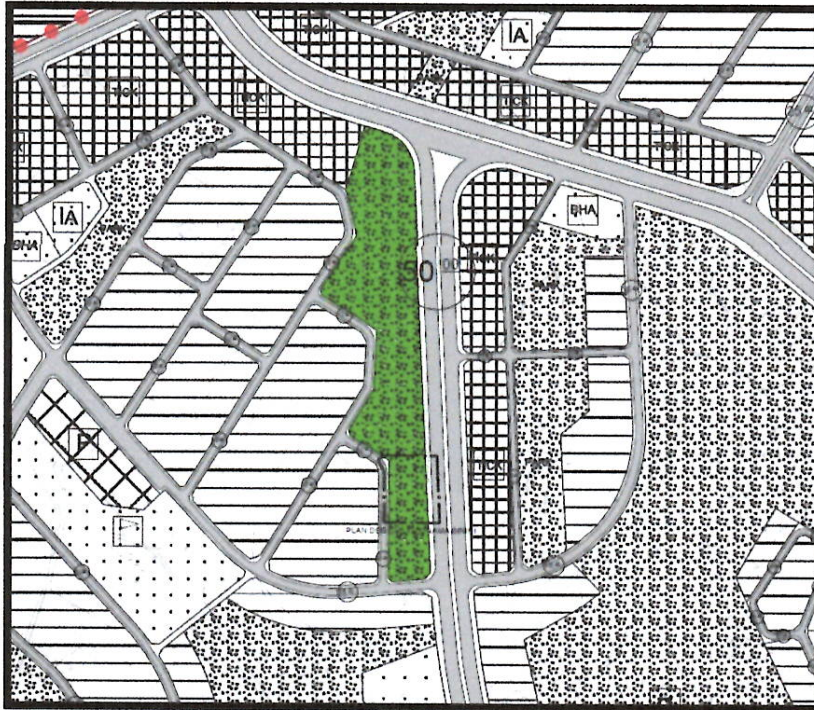
Şekil 6: Şehitkamil İlçesi Beylerbeyi Mahallesi Mevcut 1/5000 Ölçekli Nazım İmar Planı
