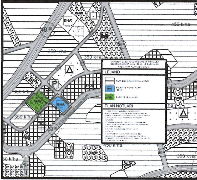
Şekil 8: Şahinbey İlçesi Küçükızıllıhisar Mahallesi Öneri 1/5000 Ölçekli Nazım İmar Planı
