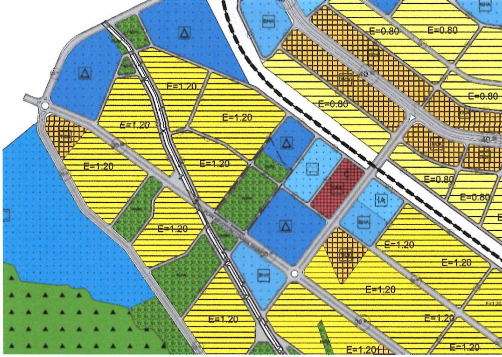
Şekil 6: Planlama Alanı Mevcut 1/5000 Ölçekli Nazım İmar Planı
