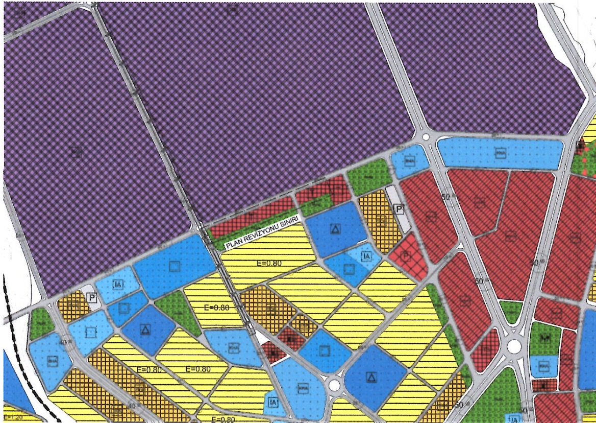
Şekil 8: Öneri 1/5000 Ölçekli Nazım İmar Planı
