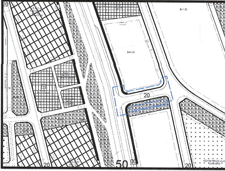
Şekil: Mevcut 1/1000 Ölçekli Uygulama İmar Planı
